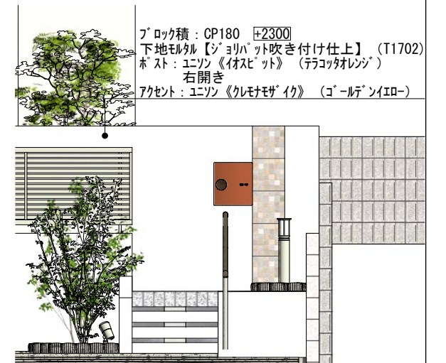
立面図 S=1/50
