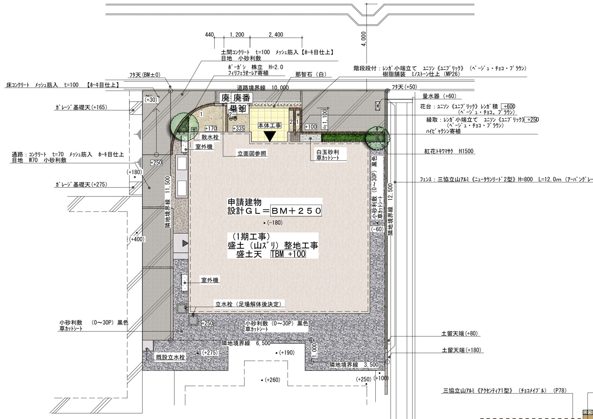
平面図 S=1/100
